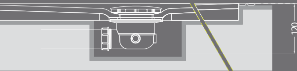
Ingombro piletta di scarico / Dimensions drain / Dimensiones de drenaje
