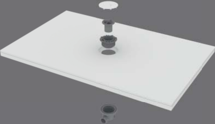
LESS / esploso del piatto doccia / exploded view of the shower / vista despiezada de la ducha
