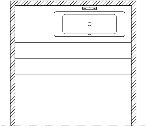
WAVE vasca medium asimmetrica con gradini / asymmetric medium bathtub with steps / bañera medium asimétrica con escalónes
