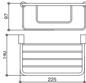
Cod. 30017CRPR Cestello rettangolare Rectangular basket
