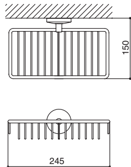
Cod. 04013CRPR Cestello rettangolare Rectangular basket
