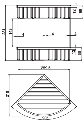
Cod. 30021CRPR Cestello doppio ad angolo Double corner basket soap holder
