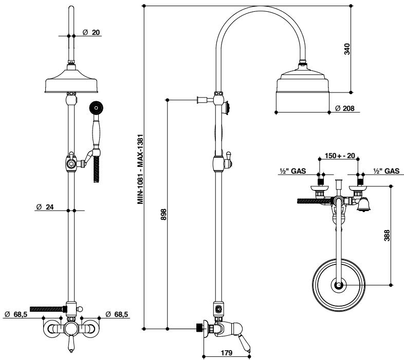
Cod. 10537CR0DPR Miscelatore doccia esterno completo di tubo doccia, deviatore, soffione diam. 208 mm. e set doccia External shower mixer with tube, diverter, diam. 208 mms. shower head and handshower set
