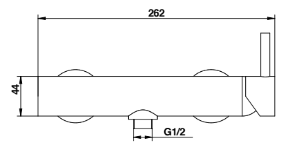
Cod. 32552CR0EPR Miscelatore doccia esterno External shower mixer
