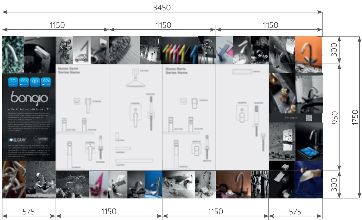
Cod. PW4 modulo da 4 pannelli lunghezza totale 3450 mm - 4 Set panel total length 3450 mms
