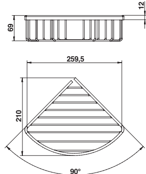
Cod. 30011CRPR Cestello singolo ad angolo Corner basket soap holder
